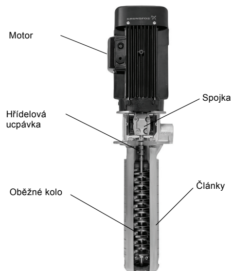
Obr. 3 Foto čerpadla MTR
