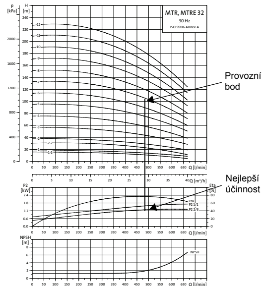
Obr. 30 Příklad provozního bodu čerpadla MTR
