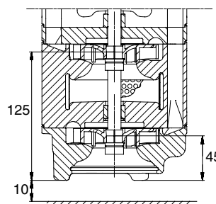
Obr. 25 Minimální vzdálenost mezi čerpadlem a nádrží
