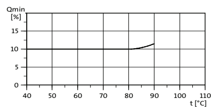
Obr. 37 Minimální průtok
