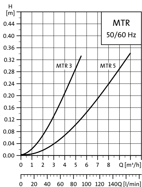
Obr. 9 Tlakové ztráty při čerpání kapaliny procházející prázdným článkem u čerpadel MTR 3 a MTR 5
