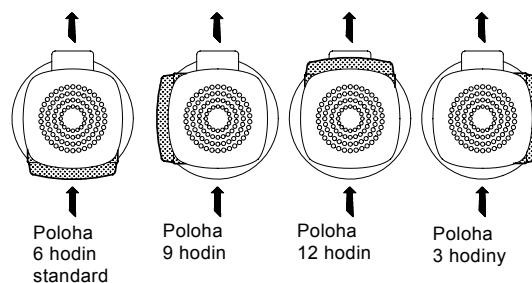
Obr. 4 Polohy svorkovnice
