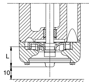
Obr. 24 Minimální vzdálenost mezi čerpadlem a nádrží
