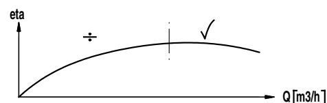
Obr. 31 Nejlepší účinnost
