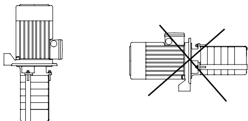
Obr. 21 Instalace čerpadla MTH
