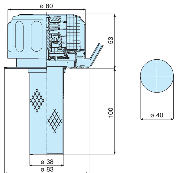
Weldable air breather caps with pre-cleaning basket Angeschweisster Belüftungsfilter mit Einfüllsieb Bouchons soudables avec panier de préfiltrage Tappi sfiato a saldare con cestello di prefiltraggio
